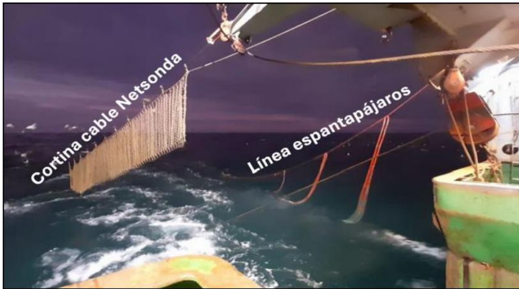
Figura 5. Embarcaciones utilizando Cortina de net sonda “Línea espantapájaros” de manera combinada. Pesquería demersal centro sur, extraído de Resolución Exenta N°250/2026. (fotografías: ATF-Chile).
